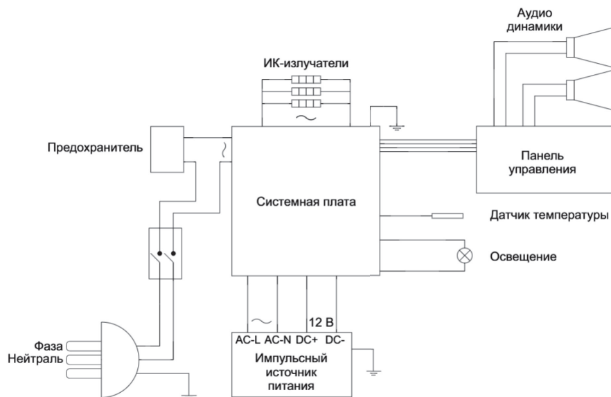
Рисунок 6. Схема подключения излучателей
