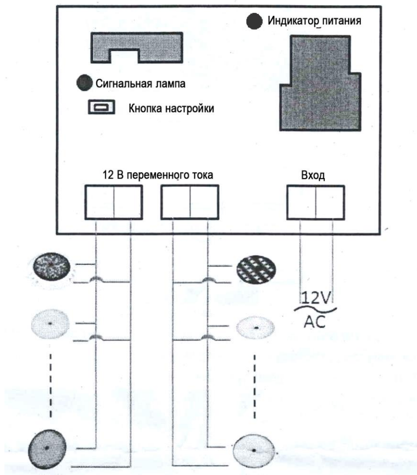
Рис. 2 Электропроводка RC01
