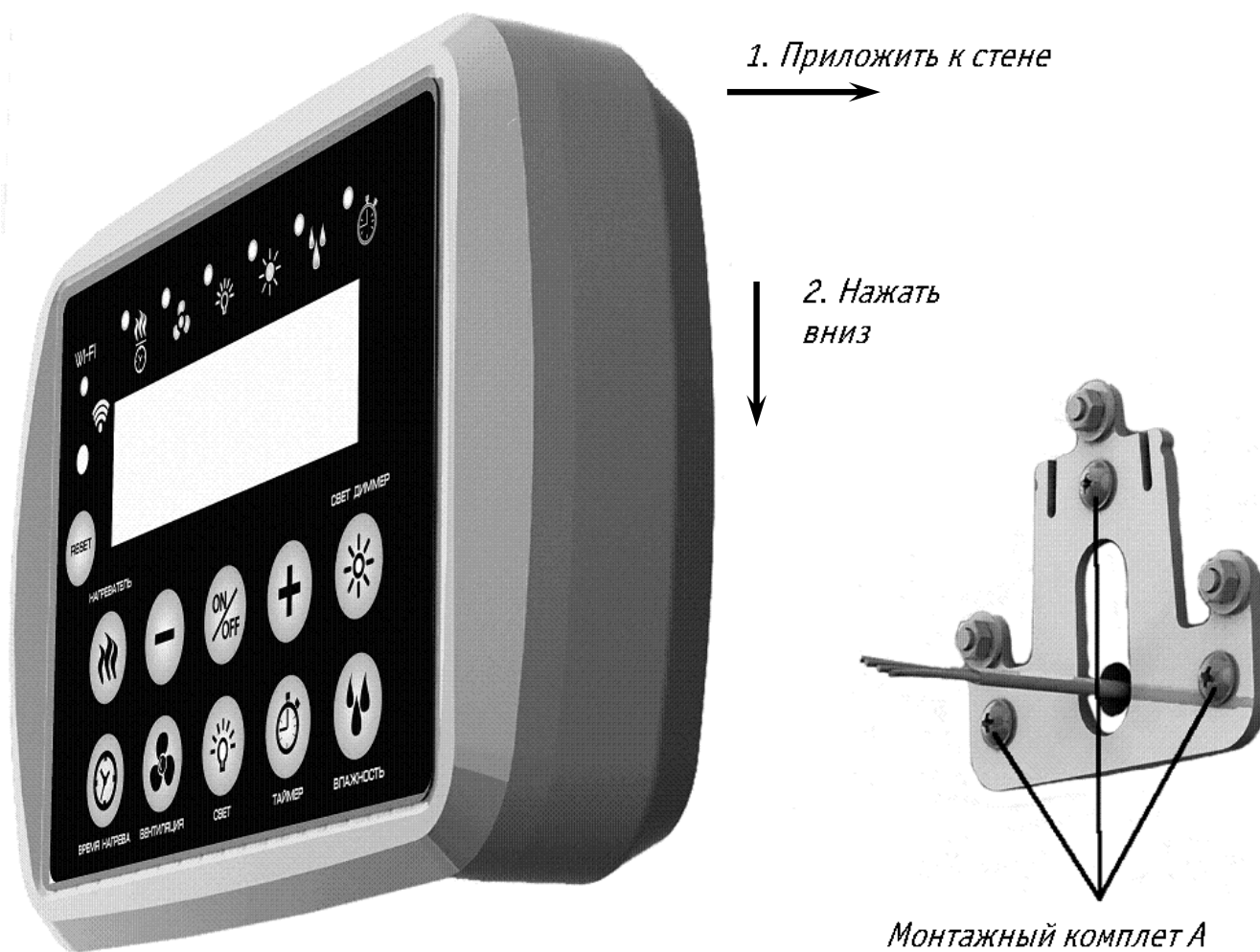
Рисунок 2. Крепление пульта управления
