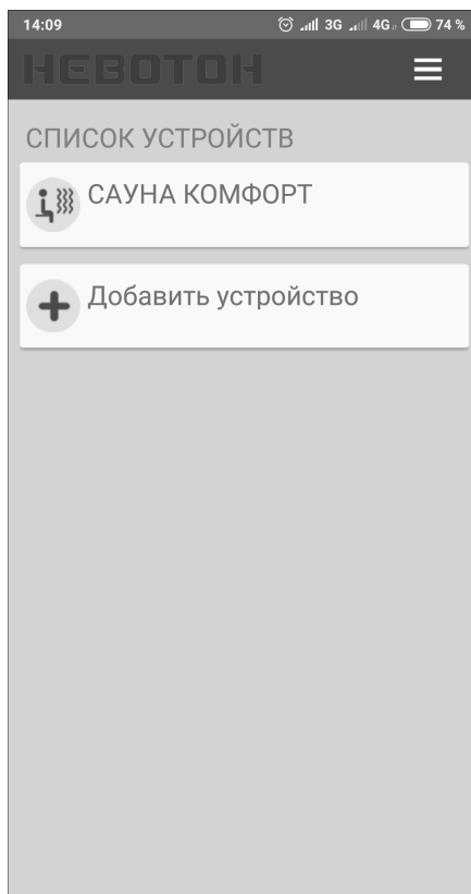
Рисунок 28 – Список устройств
