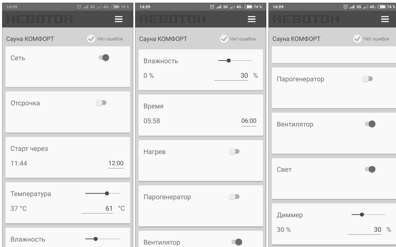
Рисунок 29 – Интерфейс Устройства в мобильном приложении
