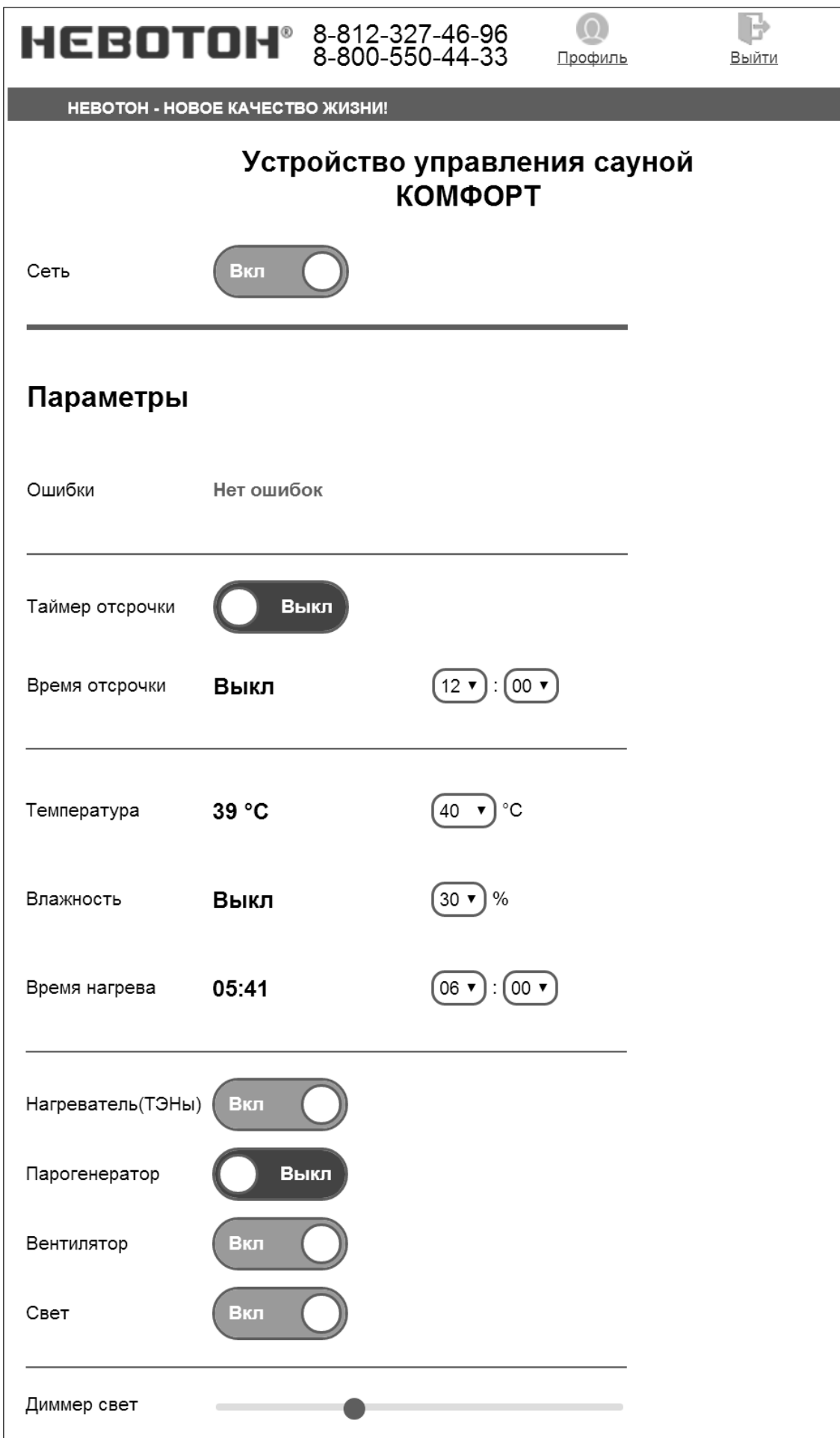
Рисунок 23. Web-интерфейс Устройства
