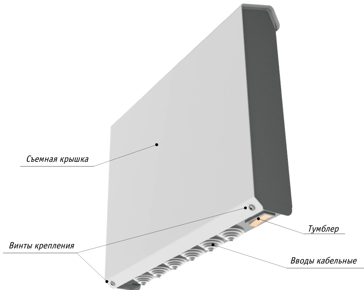
Рисунок 4. Блок коммутации
